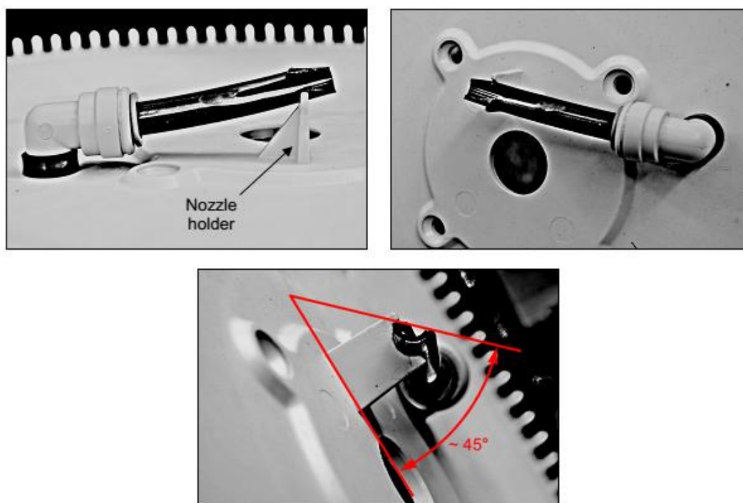
Rys. 4.5 Pozycjonowanie dyszy
