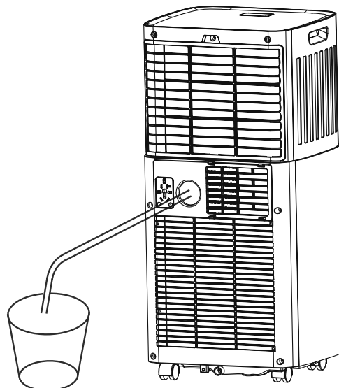
Ciągły drenaż (osuszanie)
